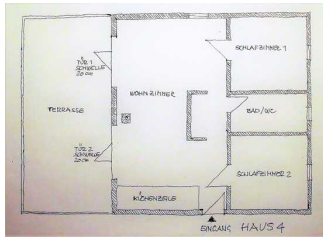
Skizze Grundriss Haus 4
